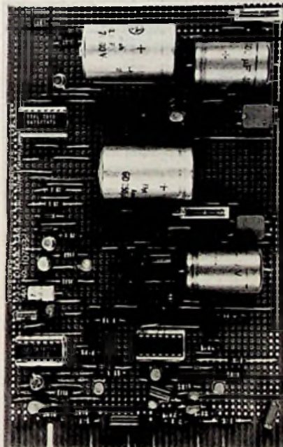
Kaart 5. ± 24 V en poort schakeling (fig. 12 en 13)
